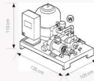
Spa-Pack filtro a sabbia (carico massimo a pavimento 260 kg/m 2 )
