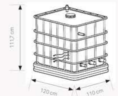
Vasca di compenso (carico massimo a pavimento 700 kg/m 2 )
